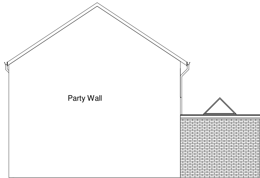
4 Side Elevation b-b 1 : 100
